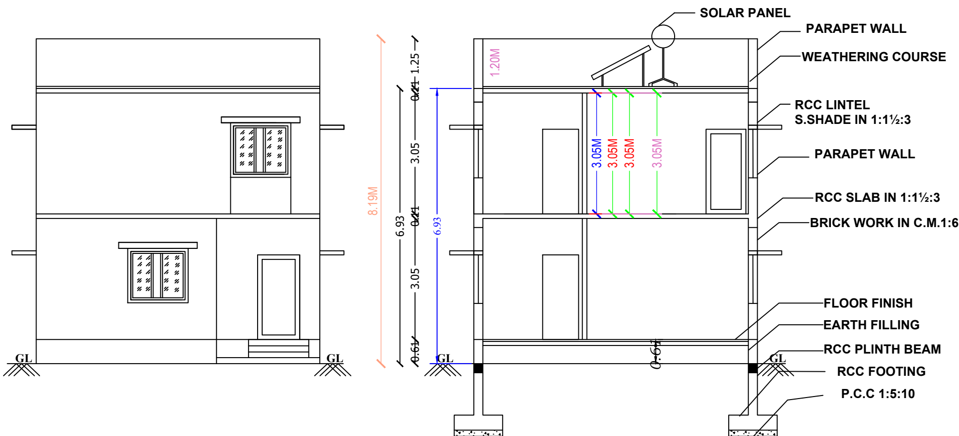
Elevation
