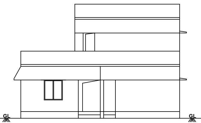
ELEVATION
