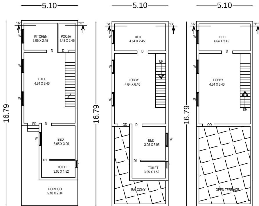
PRO. ADD S.F PLAN
