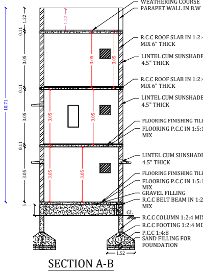
SECTION A-B
