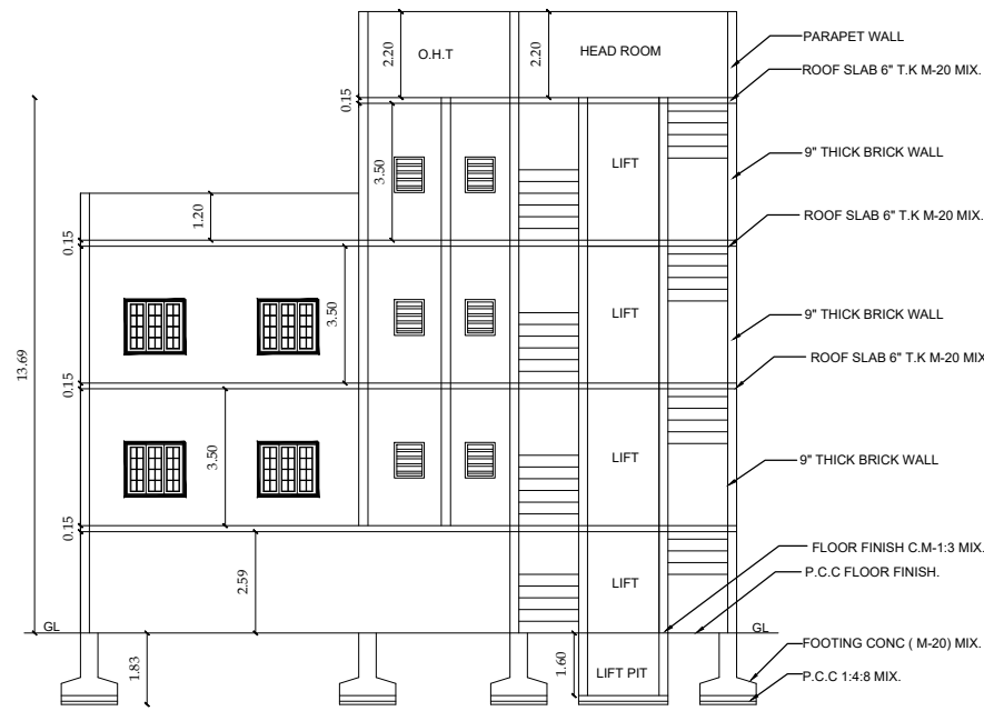
SECTION - AB
