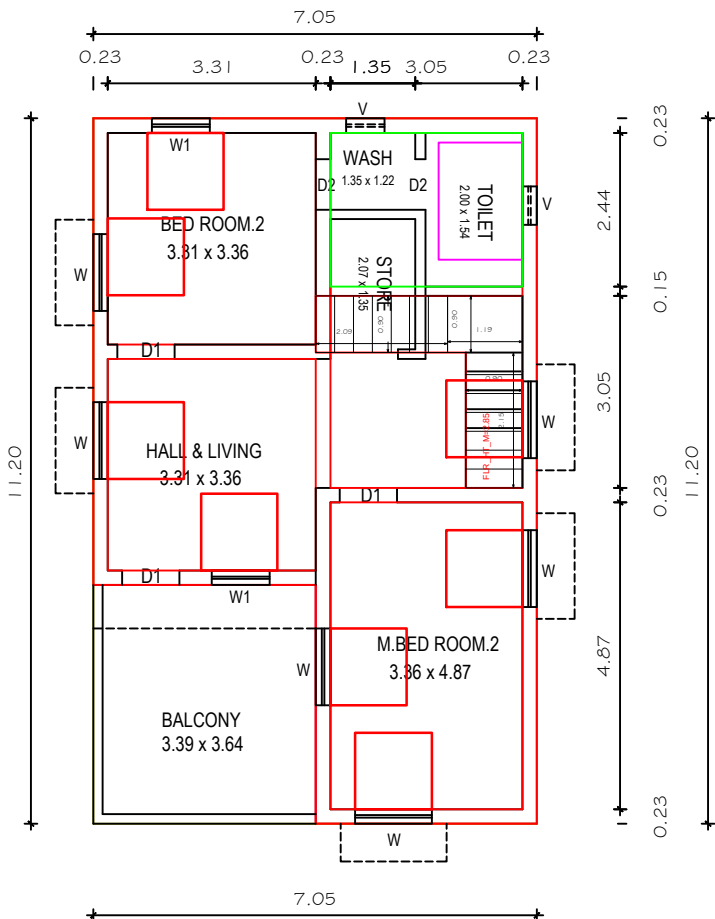
PROP.FIRST FLOOR
