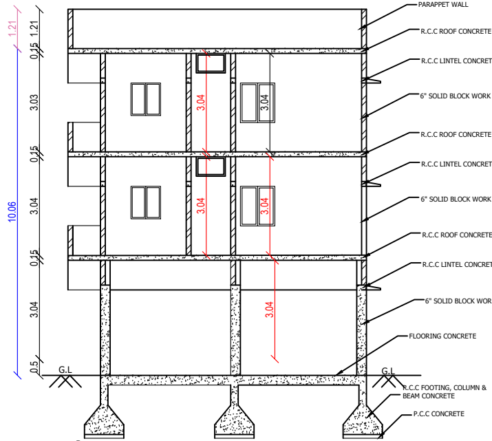
SECTION A-B
