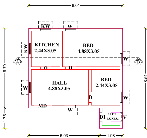
PLAN SCALE : 1 : 100
