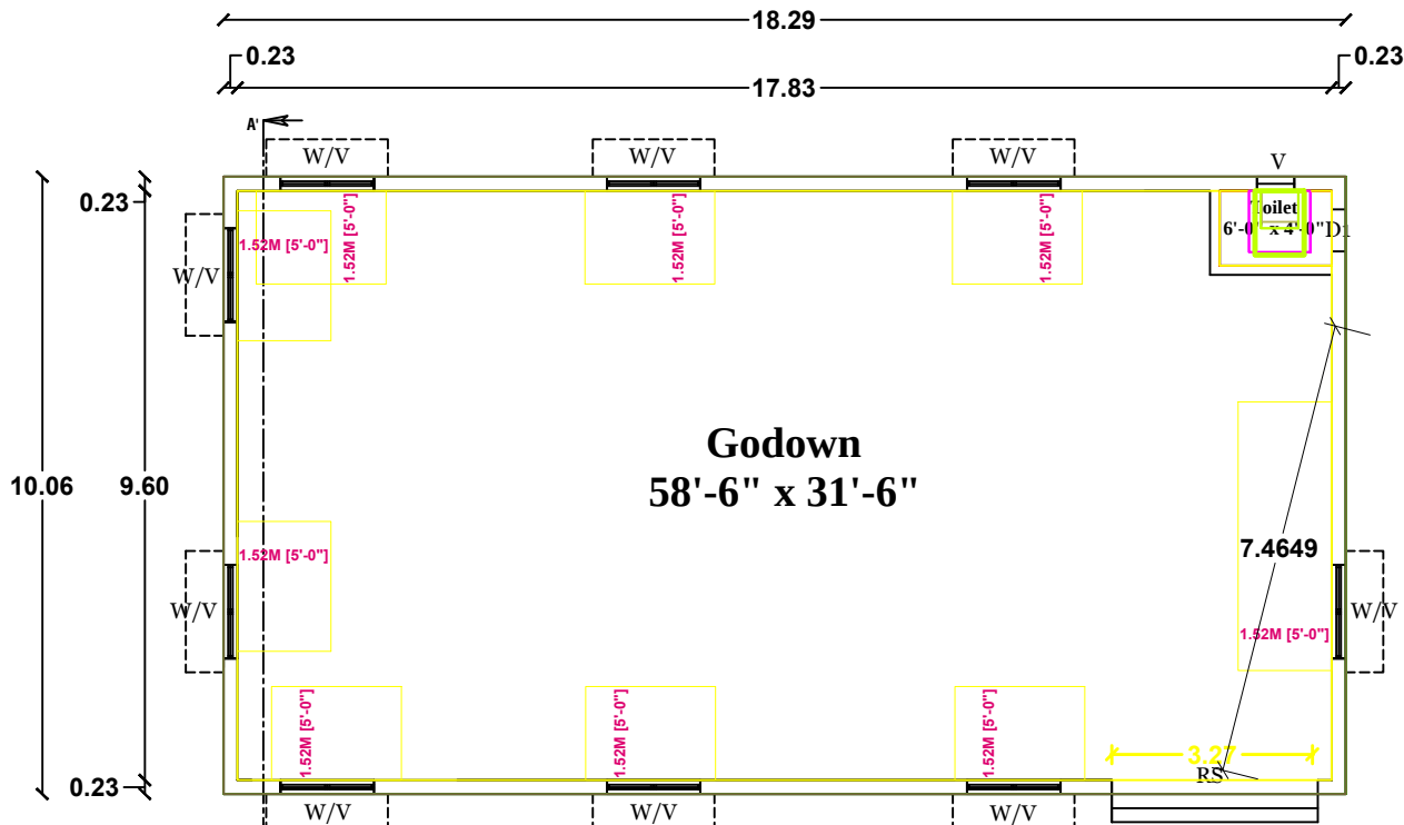
PRO.GODOWN PLAN
