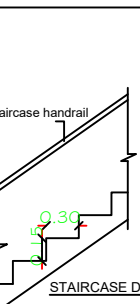
STAIRCASE DETAIL: TREAD : 0.30 m WIDTH : 0.91 m RISE : 0.15 m
