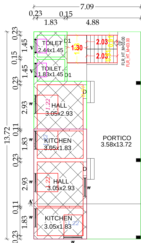
ADD. G. FLOOR PLAN
