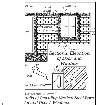
SECTION A-B
