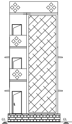
ELEVATION
