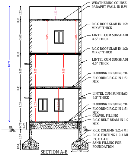
SECTION A-B
