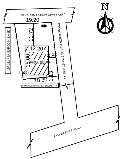
SITE PLAN(Scale 1: 400)
