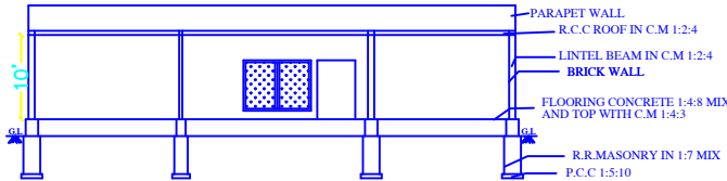
SECTION A-A
