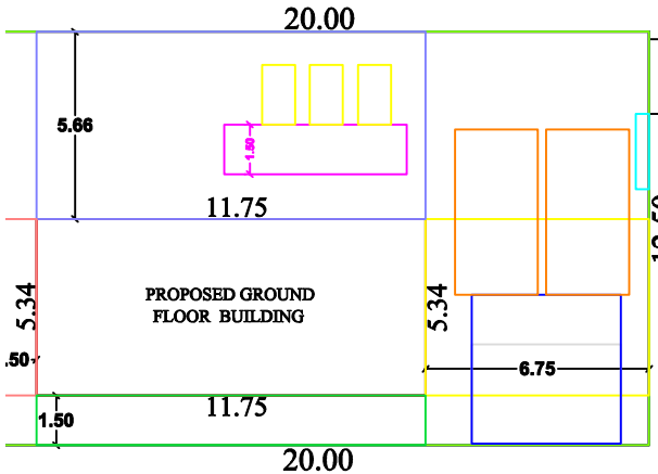
SITE PLAN ( SCALE 1:100 )
