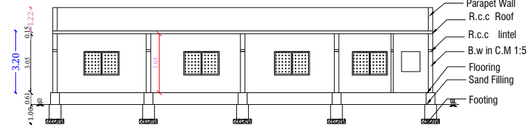
SECTION A-B
