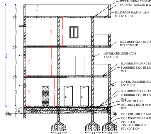
SECTION A-B
