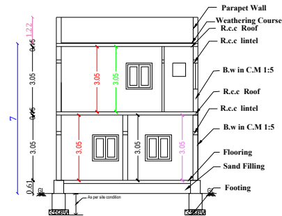
SECTION A-B
