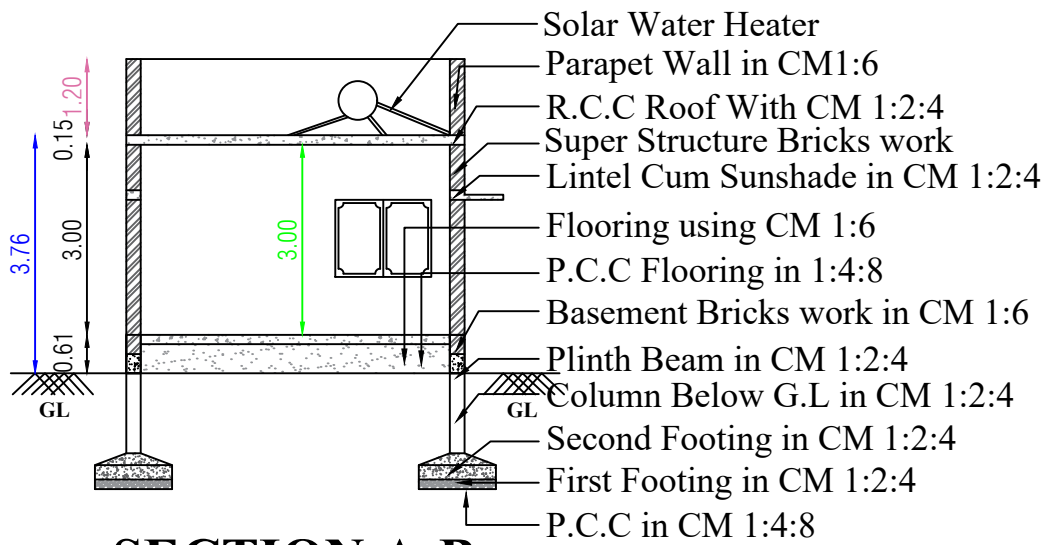
SECTION A-B
