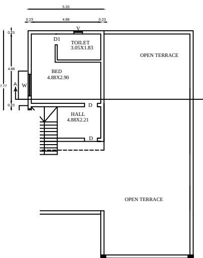
F. FLOR PLAN
