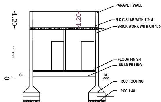
SECTION A-B
