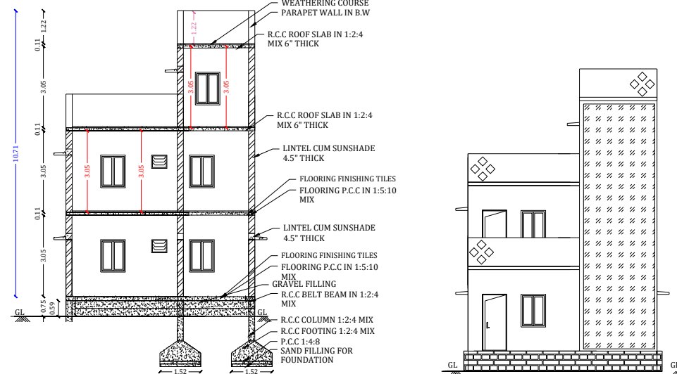
ELEVATION
