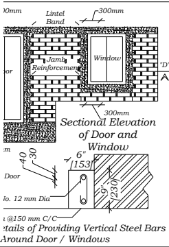
SECTION A-B
