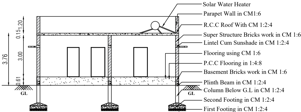
SECTION A-B
