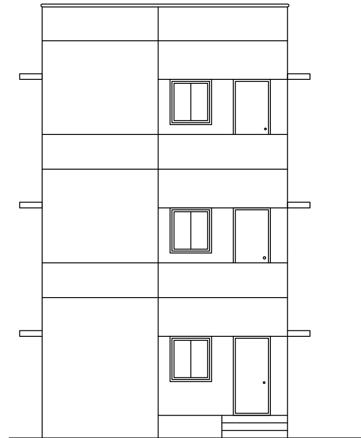
ELEVATION
