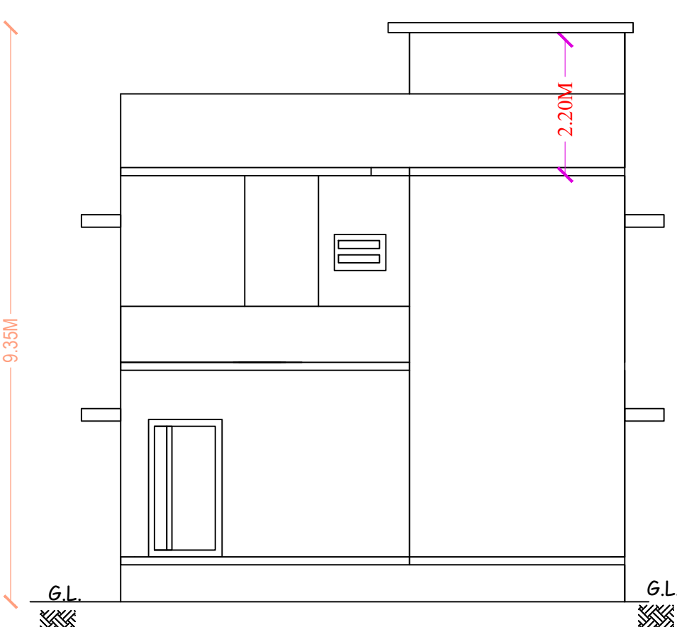
ELEVATION
