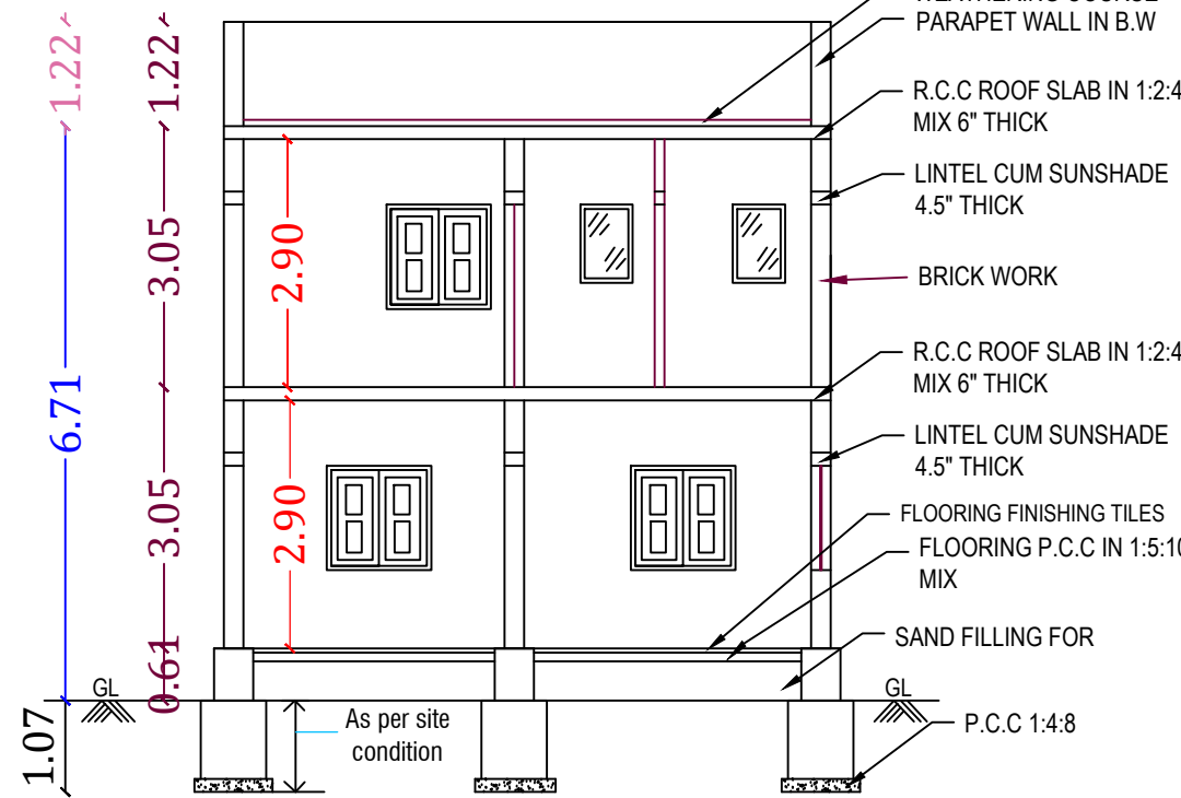
SECTION A-B
