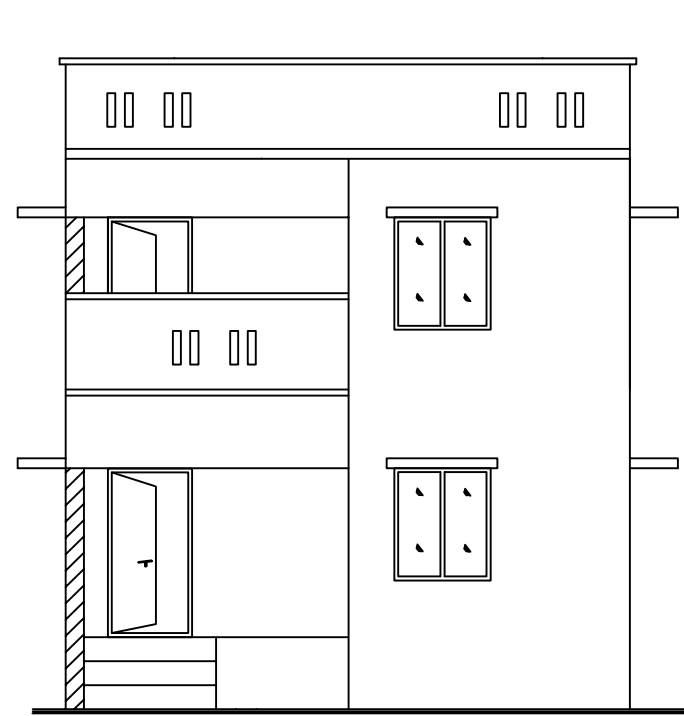
ELEVATION
