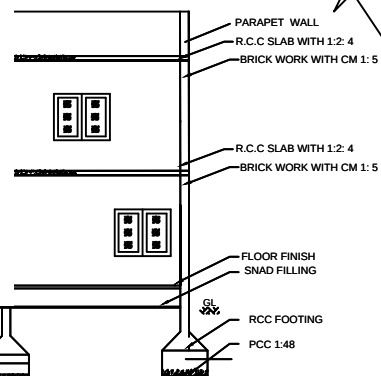
SECTION A-B
