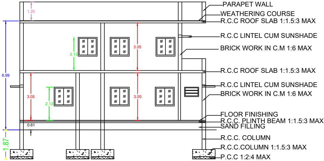
SECTION - AB
