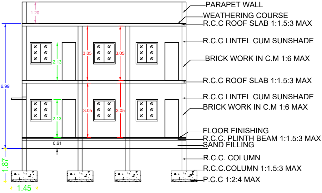
SECTION - AB
