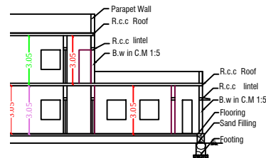
SECTION A-B
