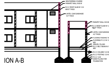
ELEVATION A-B
