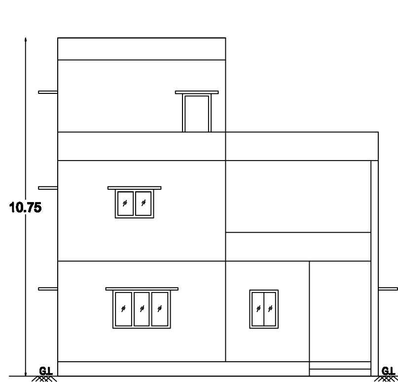
ELEVATION
