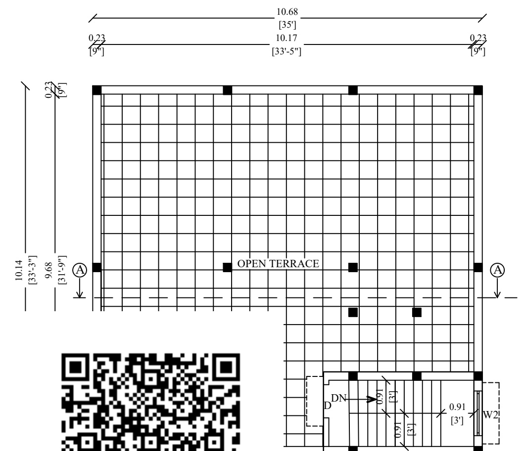
DOOR PLAN
