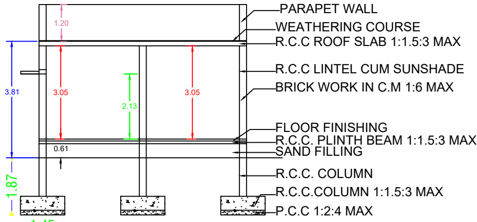
SECTION - AB
