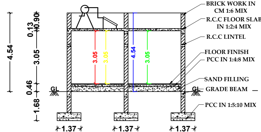
SECTION A-B
