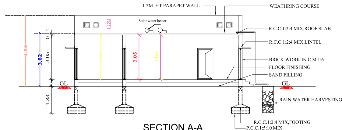
SECTION A-A
