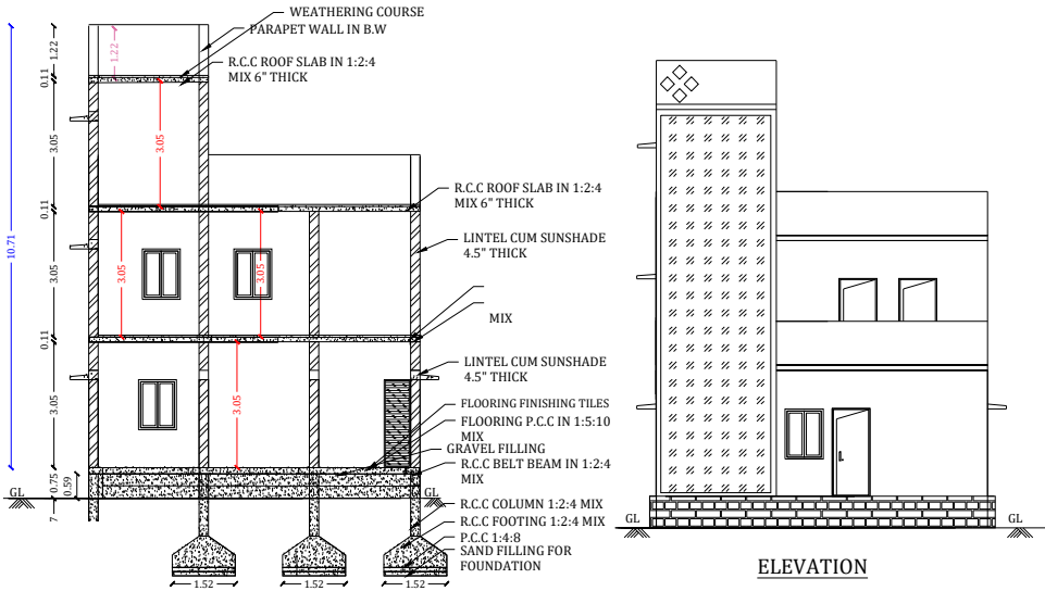
SECTION A-B
