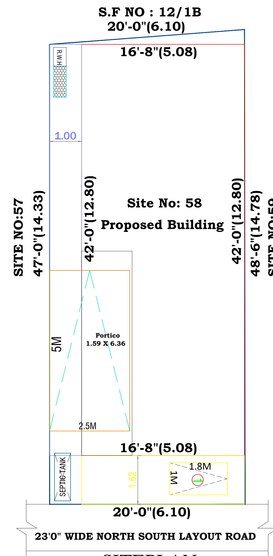
SITEPLAN
