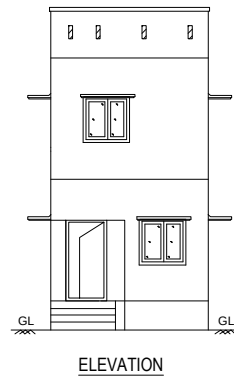
ELEVATION
