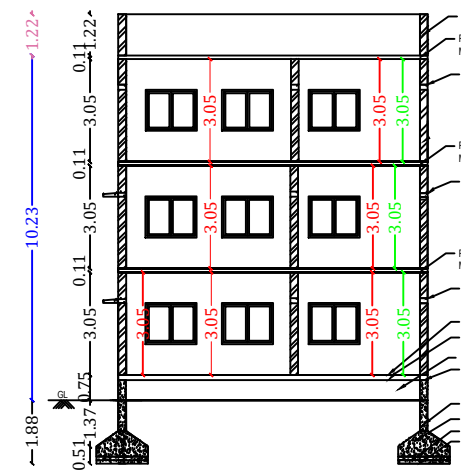
SECTION A-B
