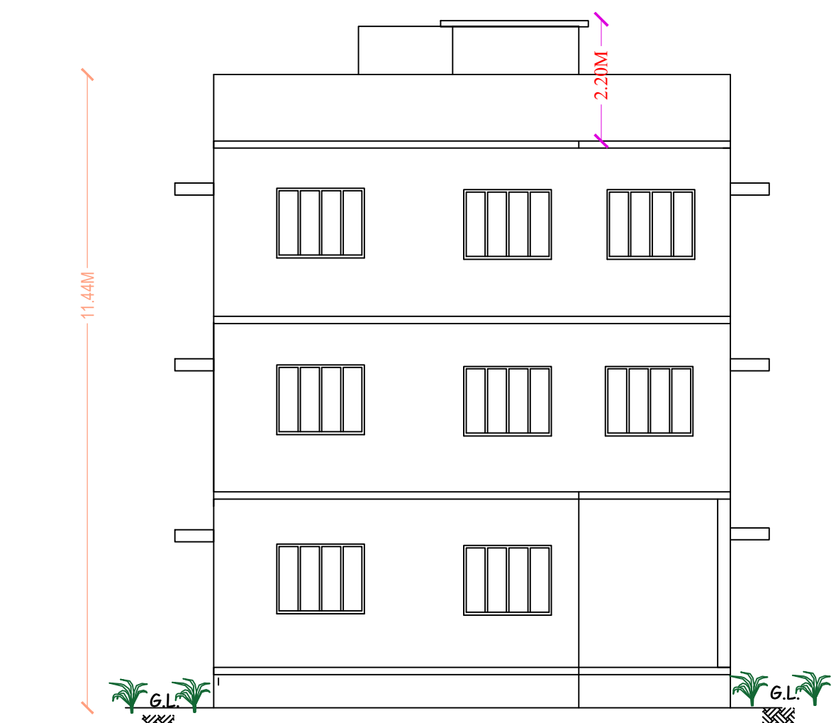
ELEVATION
