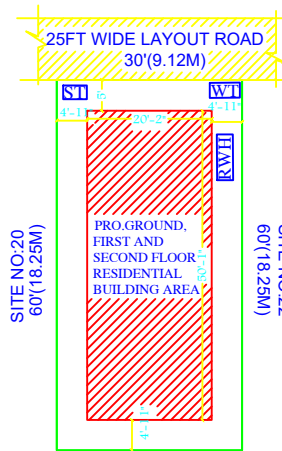
30'(9.12M) SITE NO:45 SITE PLAN
