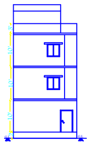
ELEVATION
