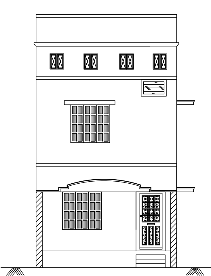
ELEVATION
