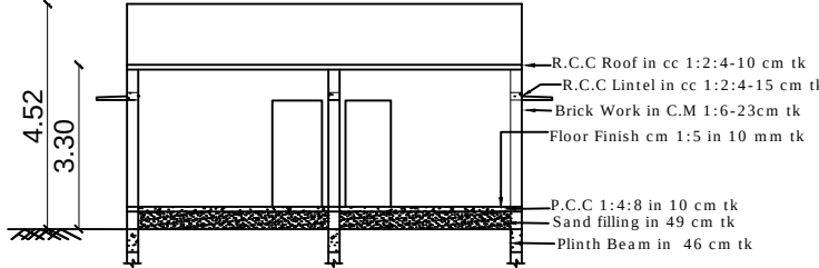
SECTION - AB
