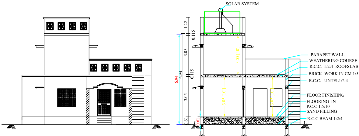
ELEVATION
