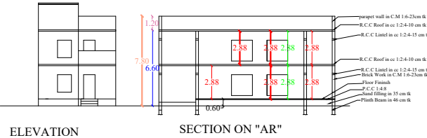
ELEVATION
