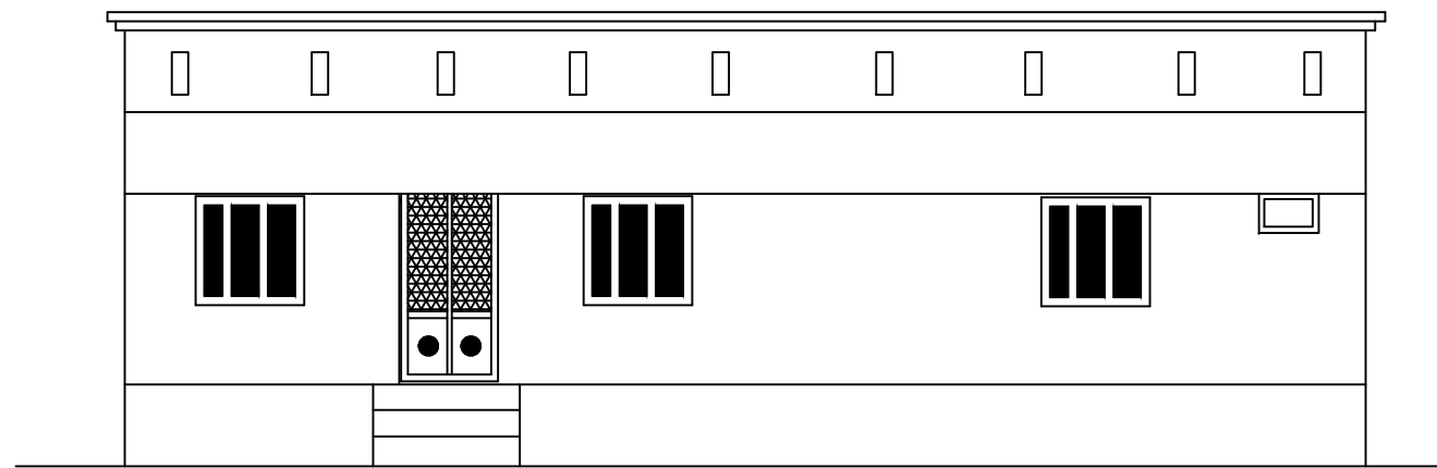
ELEVATION
