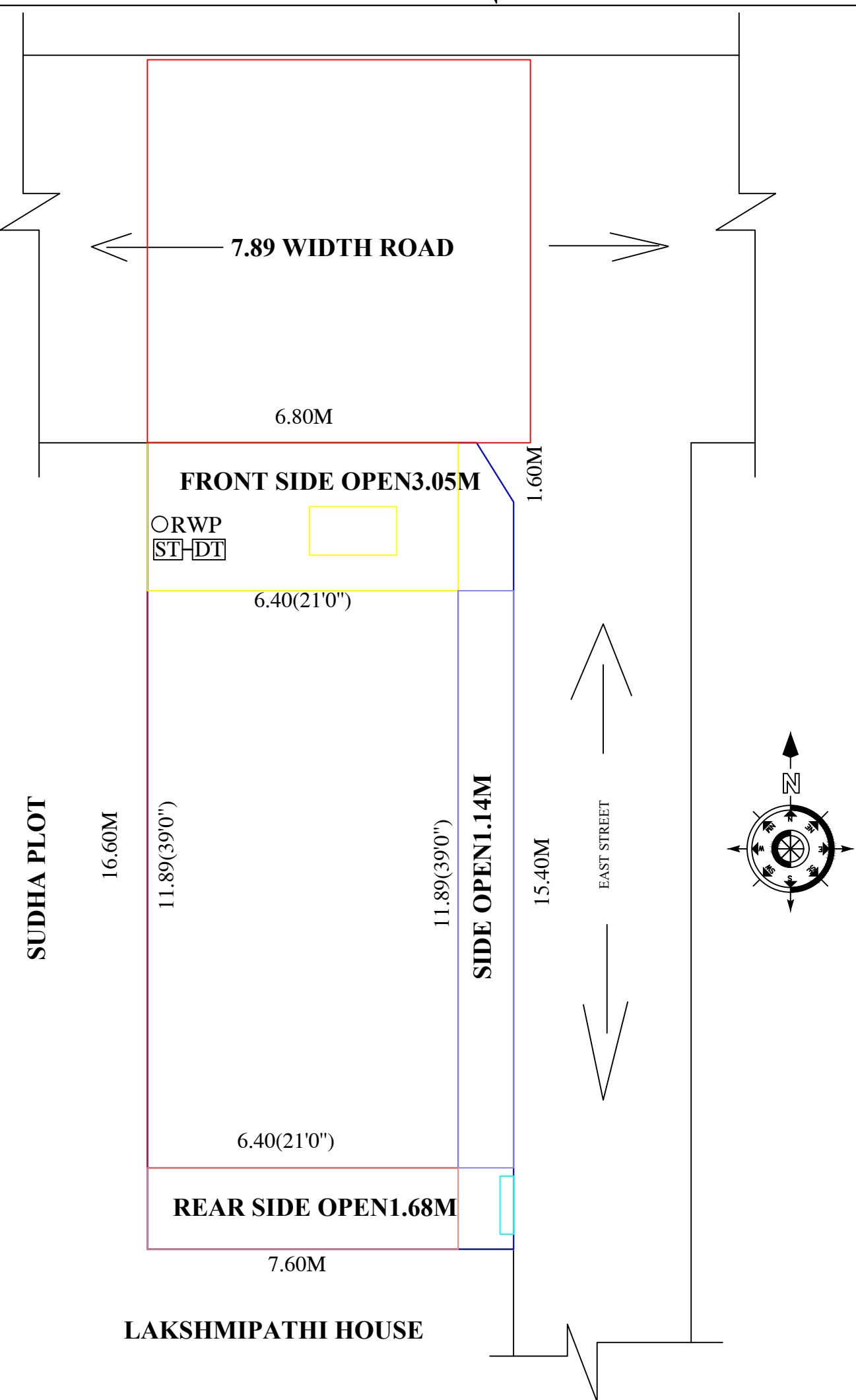
KEY MAP
